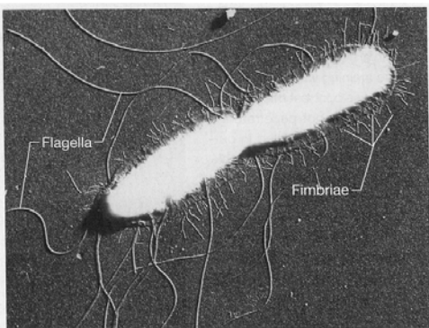
EM of Salmonella typhi
