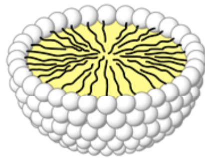
Micelle
